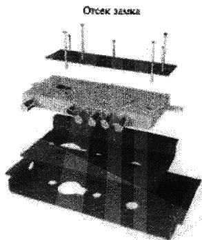
Установка вкладного замка в дверь
