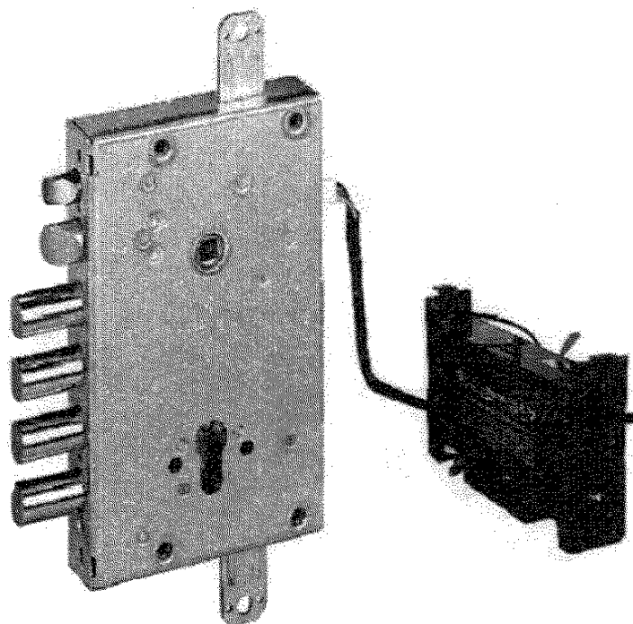
Замок с электроблокировкой
