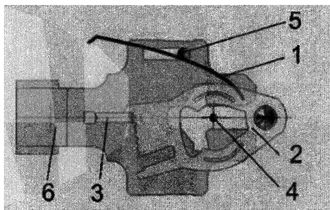
1 - возвратная пружина сувадьды; 2 - кодовая сувадьда; 3 - сувадьдная стойка; 4 - направляющий штырь ключа; 5 - направляющий штырь засова; 6 - засов.
