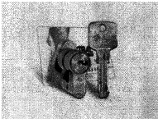
Базовый корпус типа «Евростандарт» с «перфорированным» реверсивным ключом.
