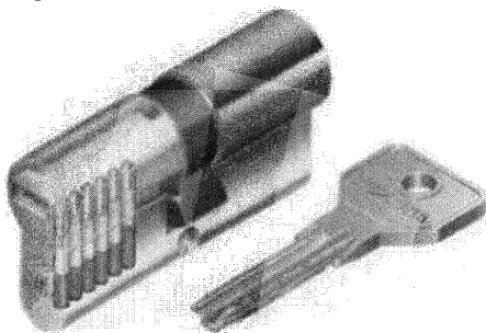
Базовый корпус типа «Евростандарт» с «перфорированным» реверсивным ключом.
