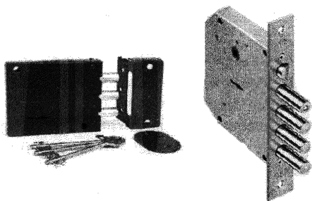
Замки: врезной и накладной с лицевыми планками
