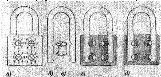
Навесной замок с шифруемой системой запирания
