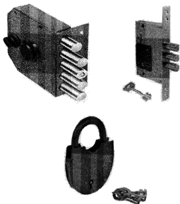
Виды сувальдных замков: Накладной, врезной, навесной
