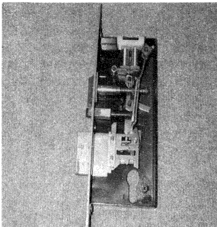
Замок с электроблокировкой
