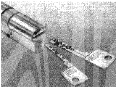
ЦМС с ключами-партнерами
