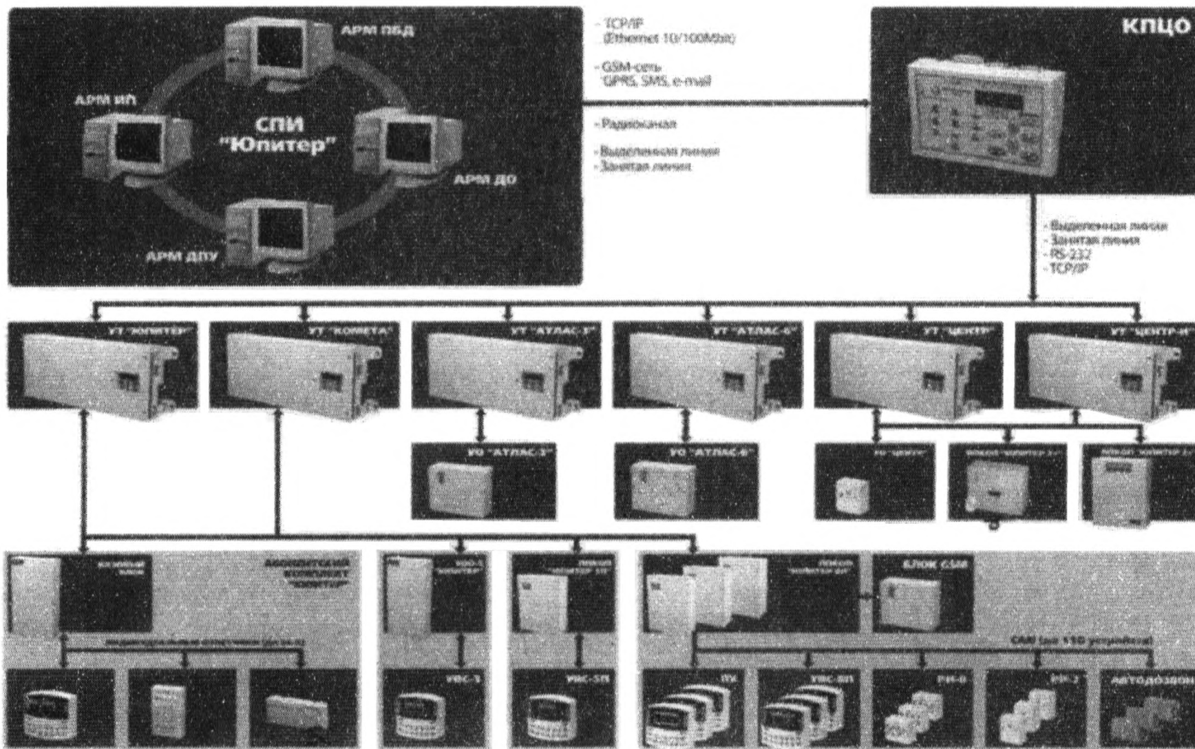
Структурная схема СПИ «Юпитер»
