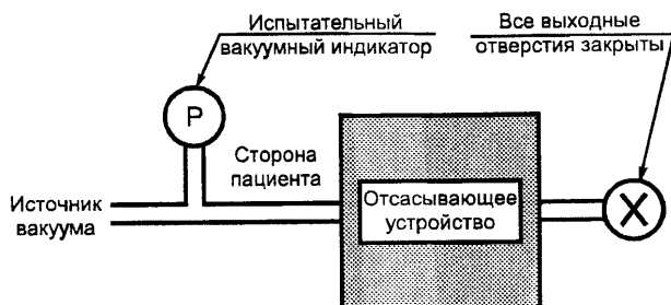
Рисунок А.5 – Схема измерения максимального допускаемого вакуума
