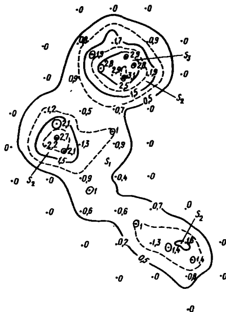
Рис. 4. Пример трансформации поля провалов в поле их плотности с учетом значений r_j и значений плотности в центрах провалов
