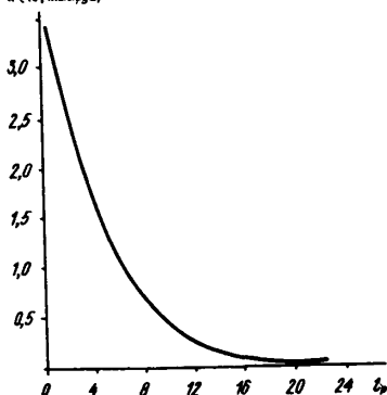
Рис. 15. Пример зависимости коэффициента эффективности противокарстовых фундаментов от расчетного пролета l_p
