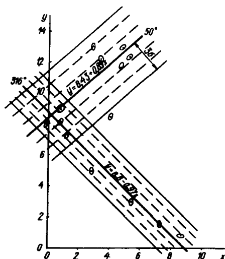
Рис. 3. Пример определения границ полос распространения провального процесса
