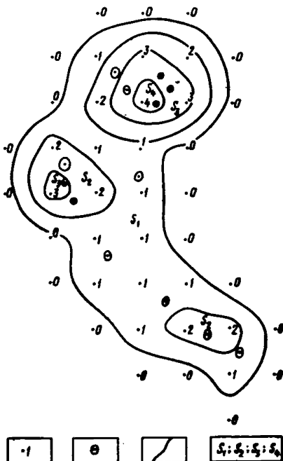
Рис. 1. Пример трансформации поля провала в поле их плотности 1 – точка измерения со значением плотности провала; 2 – карстовые провалы; 3 – границы разноточностных зон; 4 – разноточностные зоны со значениями плотности провала (1, 2, 3, 4)
