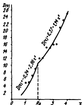
Рис. 5. Пример определения "радиуса влияния"
