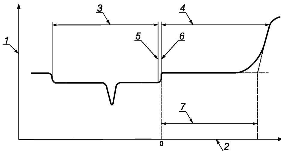
1 — изменение мощности или температуры; 2 — время; 3 — нагревание по программе (азот); 4 — изотермальный переход (кислород); 5 — переключение на изотермальный процесс; 6 — переключение на кислород; 7 — ВОИ
