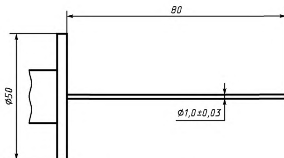
Рисунок 2 - Испытательный щуп
