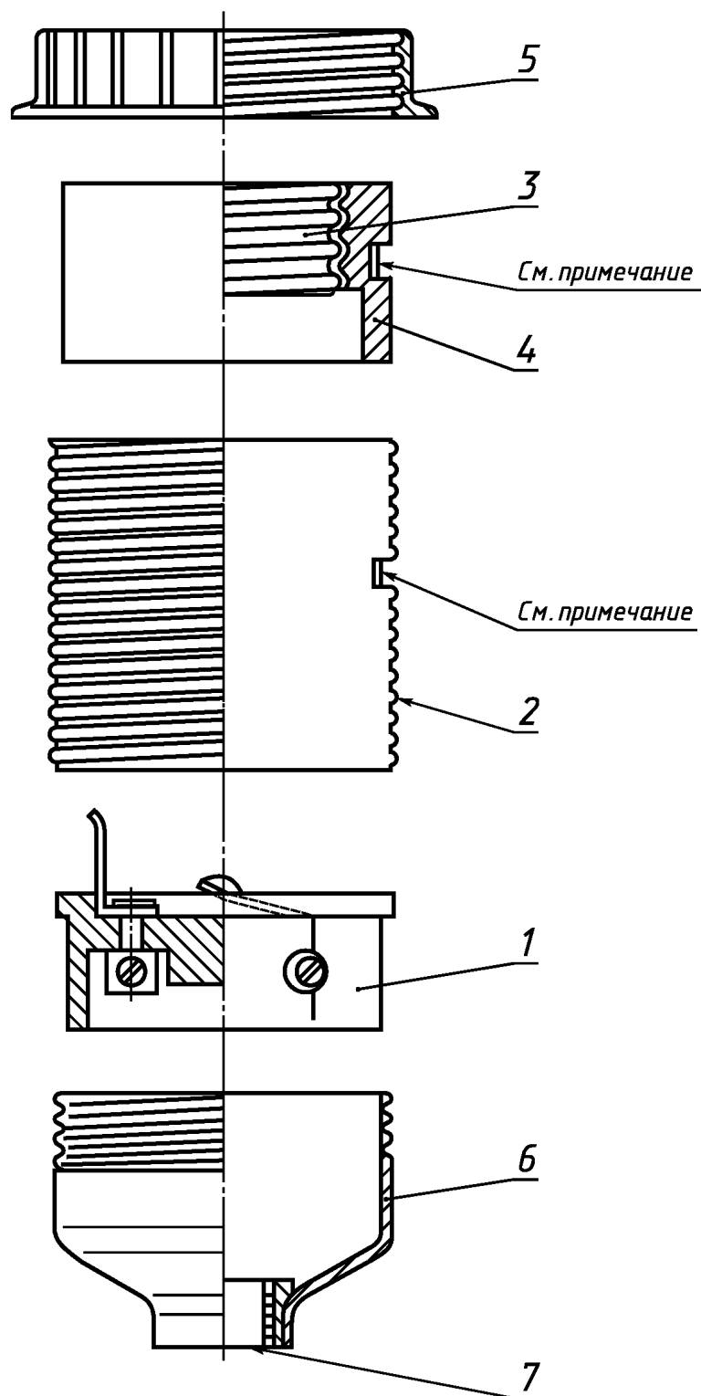
1 — сборка зажим/контакт; 2 — наружный корпус; 3 — резьбовая гильза; 4 — изолирующее кольцо; 5 — абажурное кольцо; 6 — доньшко; 7 — резьбовой ввод
