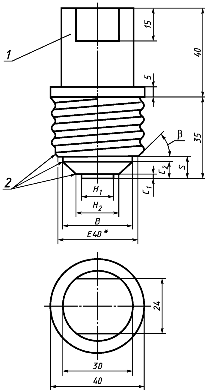
1 — твердая сталь; 2 — острые кромки притупить
