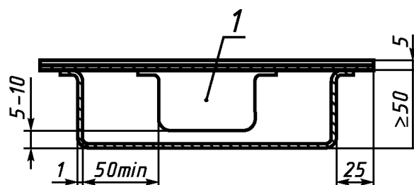
Рисунок 7 — Испытательный кожух для тепловых испытаний ПРА
