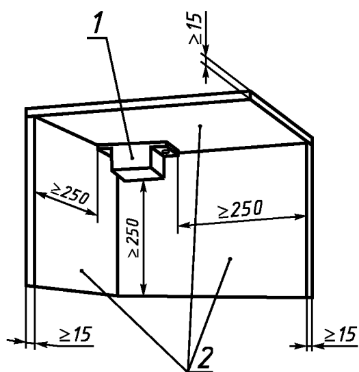
1 — ПРА; 2 — доски, покрытые матовой черной краской
