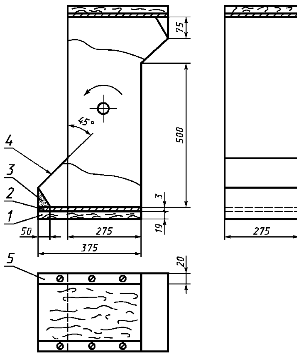
Рисунок 4 — Вращающийся барабан
