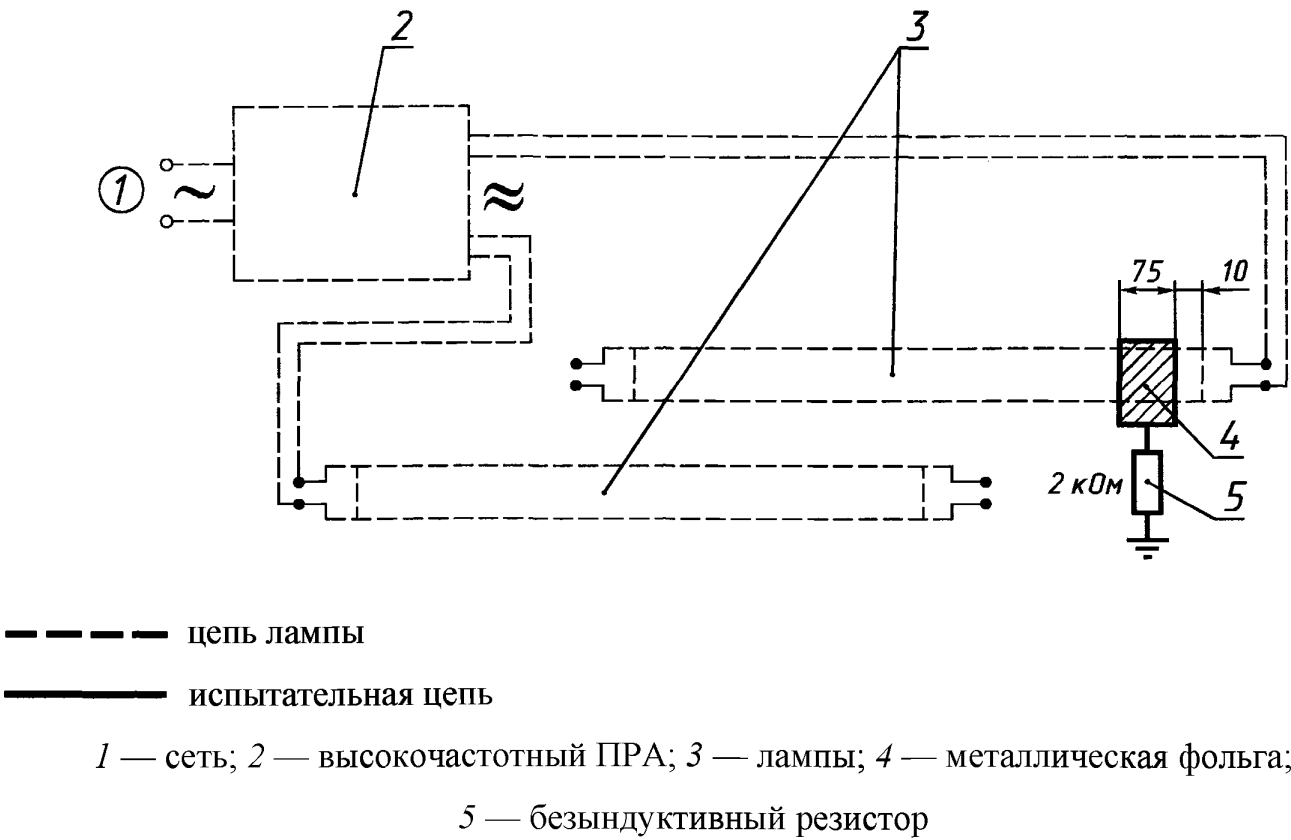
Рисунок 4 — Испытательное устройство
