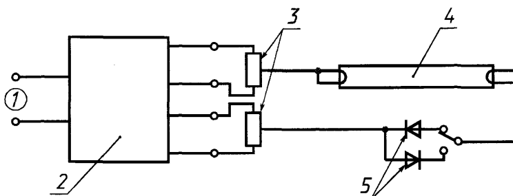
Рисунок 1 — Схема проверки выпрямляющего эффекта
