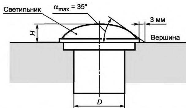
Рисунок 1 — Основные размеры, указанные в приложении А
