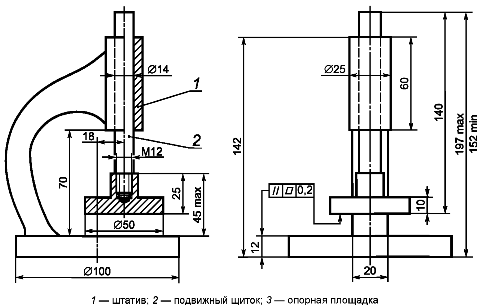
Рисунок В.1 — Приспособление для формирования опорных площадок
