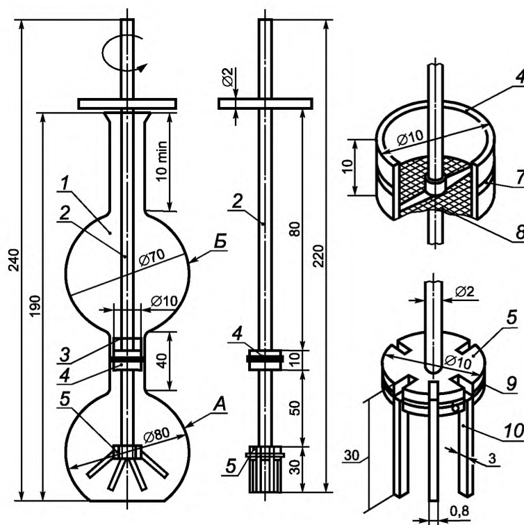
1 — основная (А) и дополнительная (Б) емкости двойной колбы; 2 — шток; 3 — метка; 4 — поршень; 5 — мешалка; 6 — перекадина; 7 — уплотнительное кольцо; 8 — сетка №063; 9 — ободок из проволоки диаметром 1 мм; 10 — лопасти
