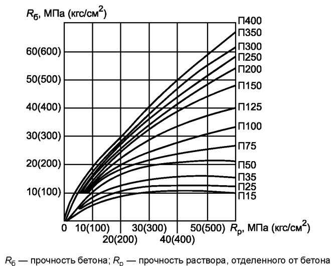
Рисунок 10 — Номограмма для определения марочной прочности крупного заполнителя
