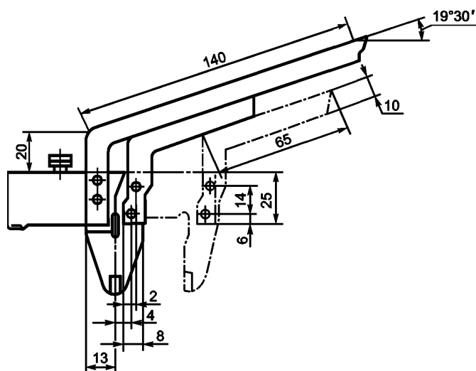
Рисунок 6 — Передвижной шаблон
