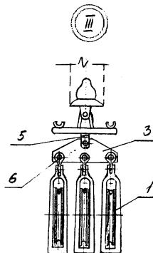
Рис. 5-3. Подъем проводов в раскаточных роликах с гирлян- дой изоляторов на промежуточную опору
