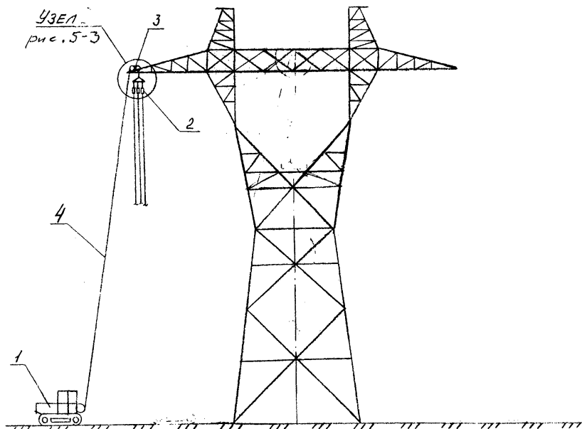
Рис. 11-1. Подъем проводов крайней фазы
