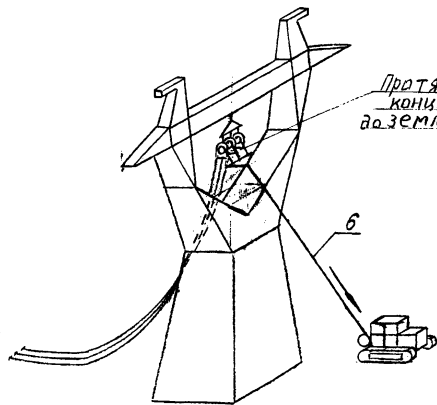
Рис. 11-2. Подъем проводов средней фазы
