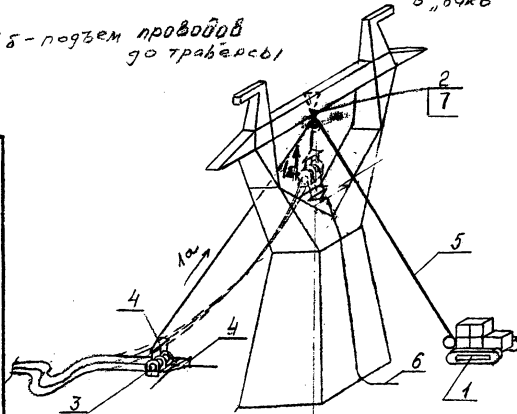
Рис. 11-2. Подъем проводов средней фазы
