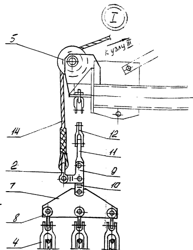
Рис. 2-1 Подъем проводов на промежуточные ПБ 500-мм опоры без гирлянд изоляторов.
