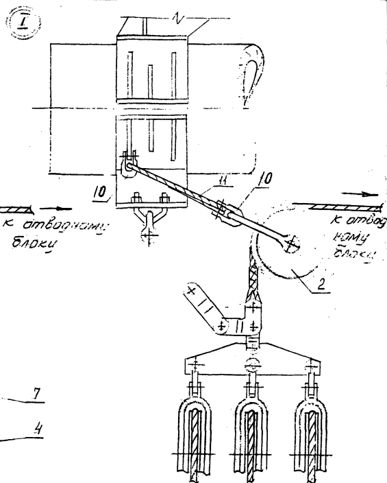
Рис.13-1. Схема подвеса проводов в раскаточных роликах на промежуточной опоре типа РБ 500-1
