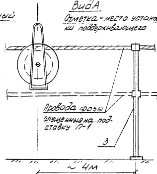
Рис. 26-1. Перекладка проводов на промежуточной опоре типа ПБ с опусканием на землю
