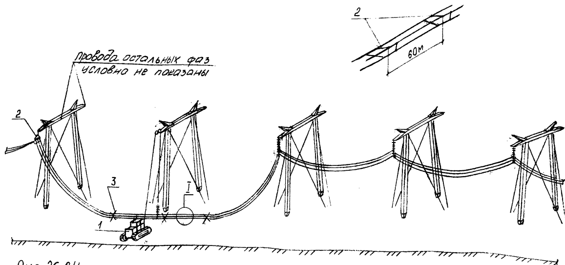
Рис. 26-24 Установка дистанционных распорок при перекладке проводов с опусканием на землю.
