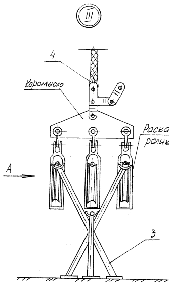
Рис. 26-1. Перекладка проводов на промежуточной опоре типа ПБ с опусканием на землю
