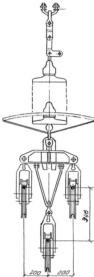
Рис. 0-5 Ширянда поддерживающая одноцелная для промежуточно-угловых опор (по типовому проекту ДП ЭСП 3516тм, альбом IV)
