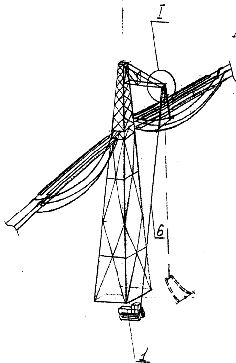
Подъем поддерживающей гирлянды шлейфа
