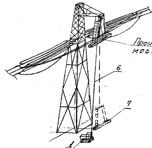
Подъем монтажной люльки для монтажа полупетель шлейфа
