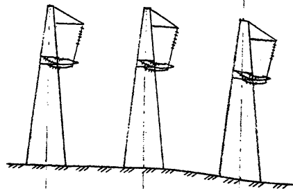
Схема расположения проводов шлейфов на анкерно-угловых опорах
