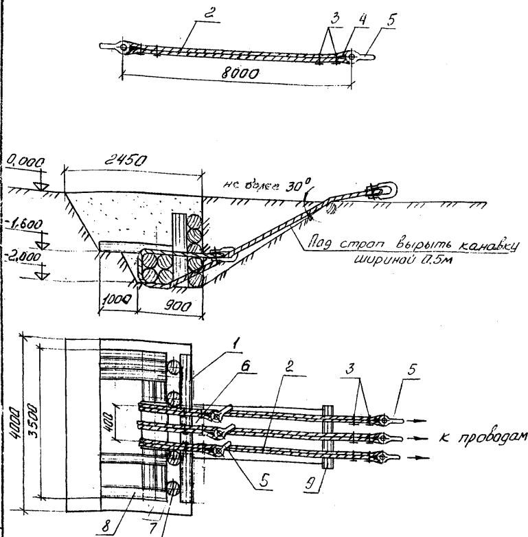
Рис. 37-1. Якорь
