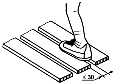
Рисунок 10 — Ширина зазоров на поверхностях наклоном до 45°
