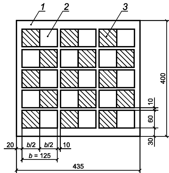
1 — фрагмент изделия; 2 — облицовочная плитка; 3 — часть плитки (образец для испытаний)
