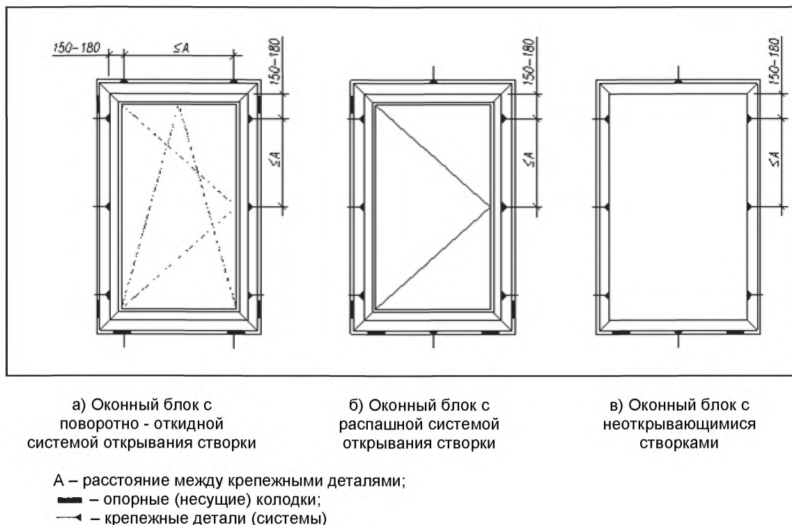
Рисунок Г.3 – Примеры расположения опорных (несущих) колодок и крепежных деталей в одностворчатых оконных блоках
