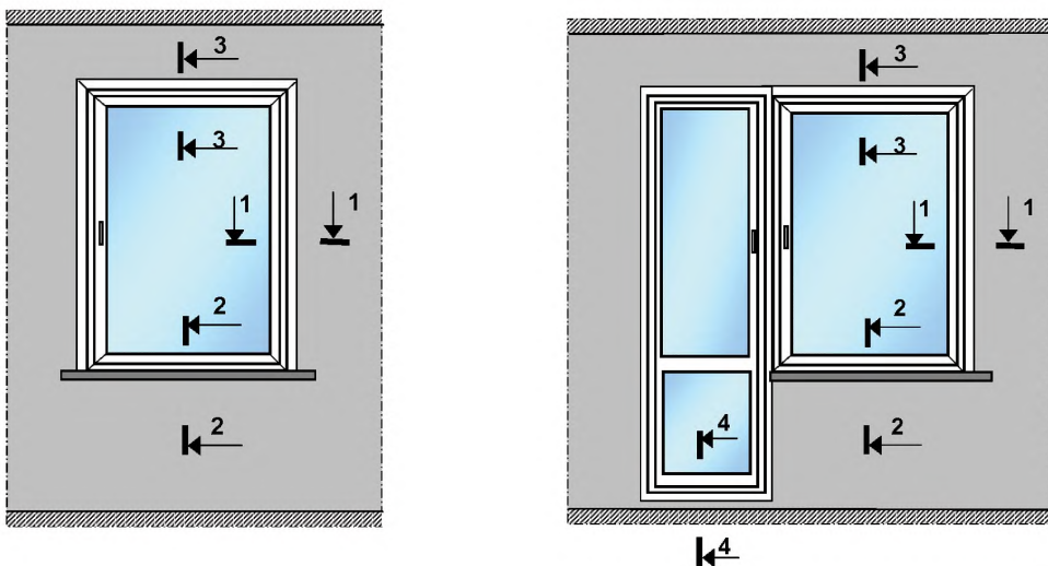
1 — горизонтальное сечение; 2, 3, 4 — вертикальные сечения а) оконный блок б) балконная дверь Рисунок Д.1 — Схема расположения сечений для проверки температурного режима узлов примыканий оконных блоков к наружным стенам:
