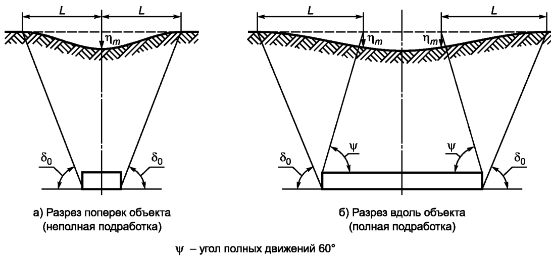
Рисунок Р.1 — Основные параметры мульты сдвижения
