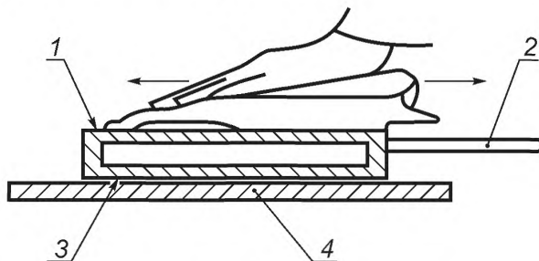
1 — поверхность А; 2 — тефлоновая ручка; 3 — поверхность В; 4 — фторопласт
