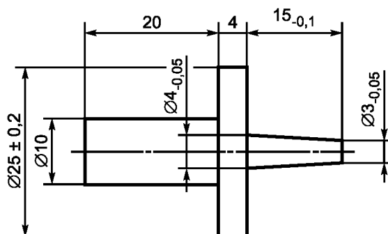
Рисунок 2 — Испытательный щуп
