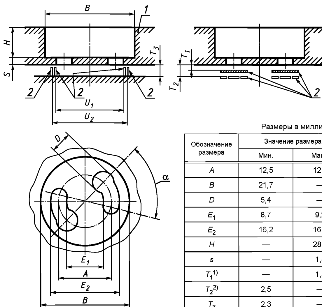
Вариант расположения контактов
