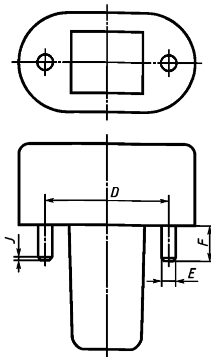
Рисунок 24 — Испытательный цоколь для испытания патронов G23 и GX23 по разделу 13
