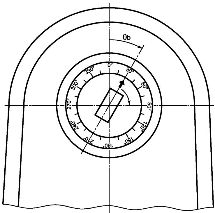
Рисунок 12b — Пример шкалы КОЛЛИМАТОРА ПУЧКА: указатель на дочернюю систему (КОЛЛИМАТОР ПУЧКА), шкала на материнскую систему (ШТАТИВ), видимые из ИЗОЦЕНТРА (см. 2.1.6.2 и раздел 3)
