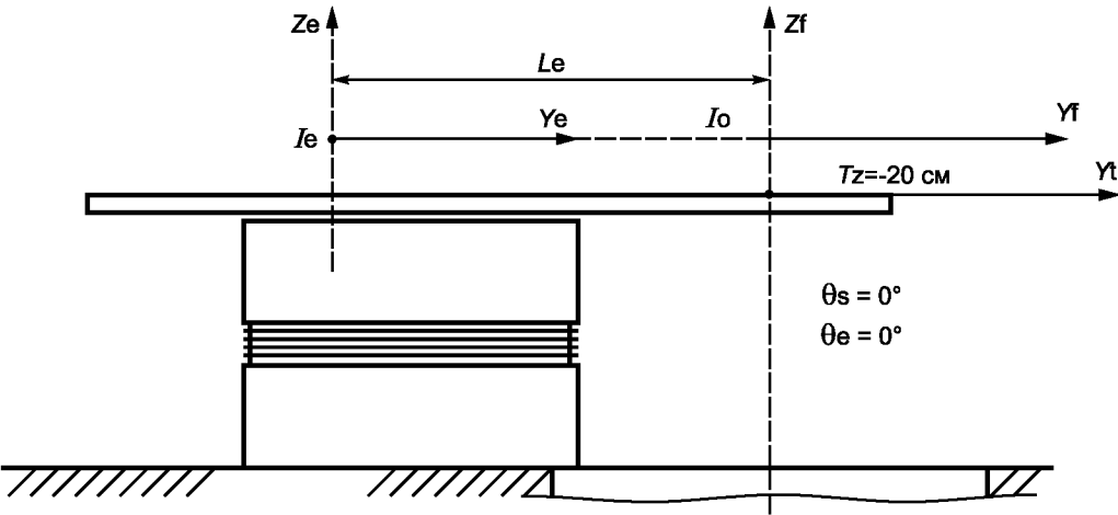
Рисунок 11а — Дека СТОЛА для ПАЦИЕНТА находится под ИЗОЦЕНТРОМ на расстоянии Tz = -20\text{ см} (см. 2.8 и 2.9)
