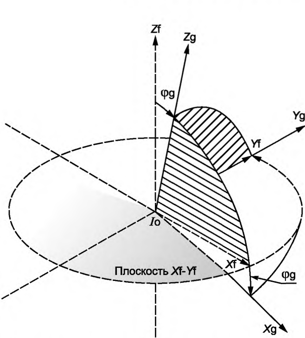
Рисунок 4 — Поворот на угол \varphi_g = 15^\circ системы координат ШТАТИВА X_g, Y_g, Z_g в неподвижной системе координат X_f, Y_f, Z_f (см. 2.3)
