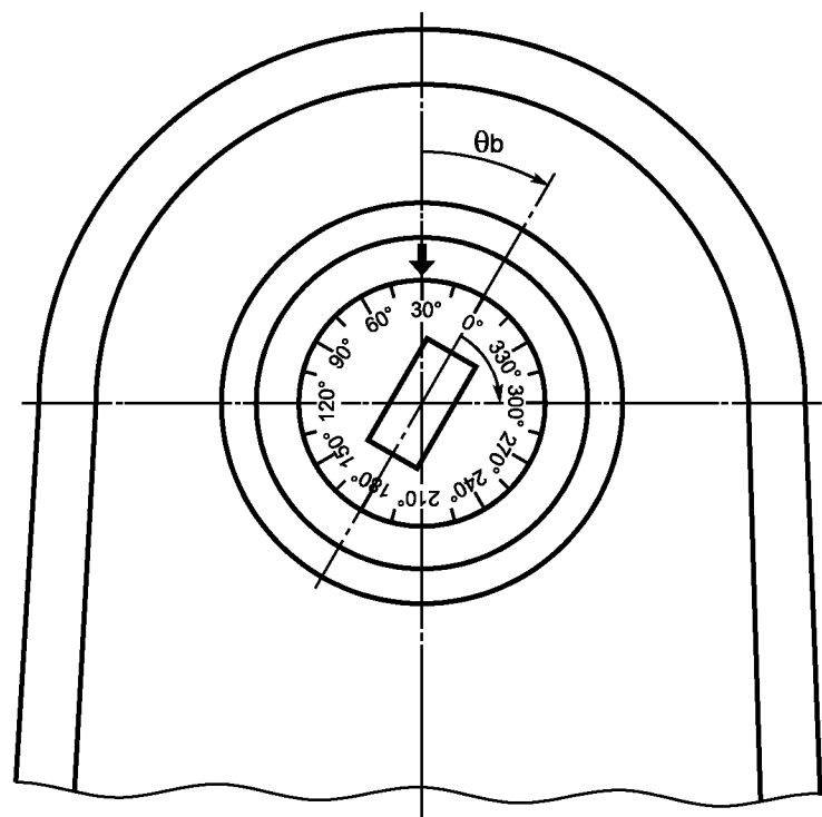
Числовая индикация угла поворота КОЛЛИМАТОРА ПУЧКА: 30°
