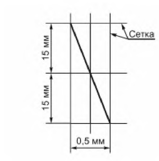
Рисунок 109 – Проверка прямоугольности системы координат (см. 51.108.4.1)
