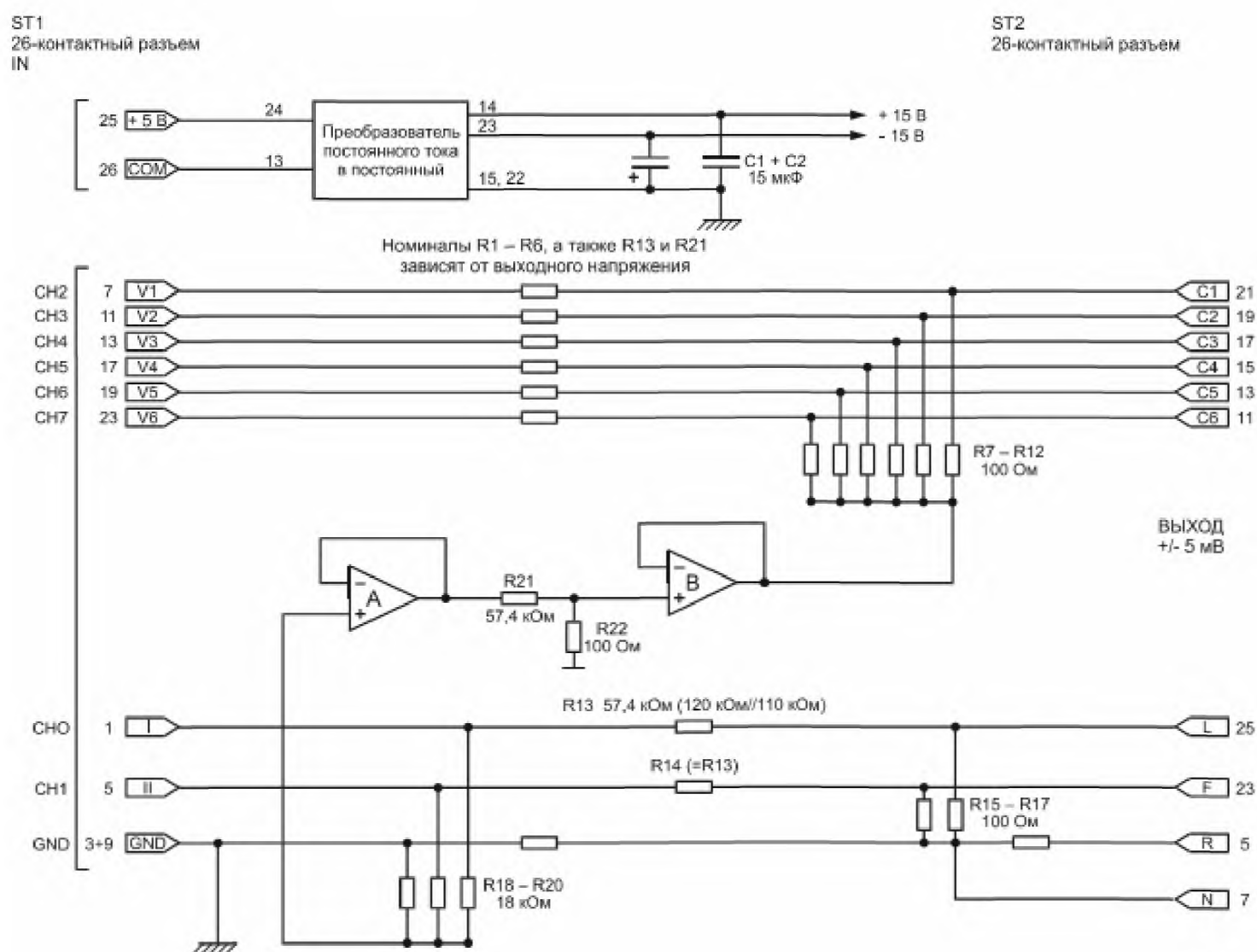
Рисунок II.2 – Пример схемы предварительной обработки ЭКГ-сигналов
