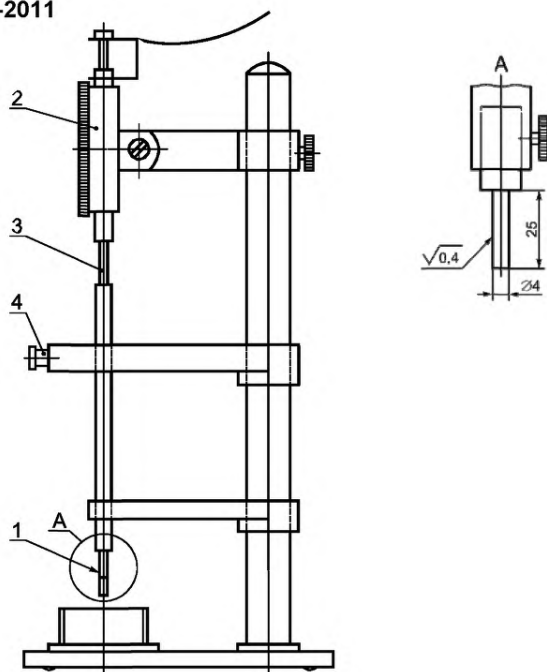
1 — индентер с иглой; 2 — цифровой индикатор; 3 — шпиндель; 4 — блокировочное устройство
