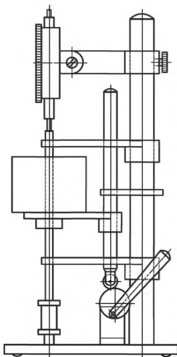
Рисунок 6 — Устройство для испытания на деформацию сжатия
