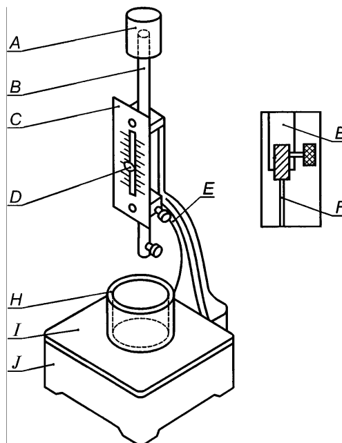
Рисунок 1 — Схема прибора Вика
