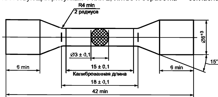
Рисунок 1 — Образец с короткой головкой
