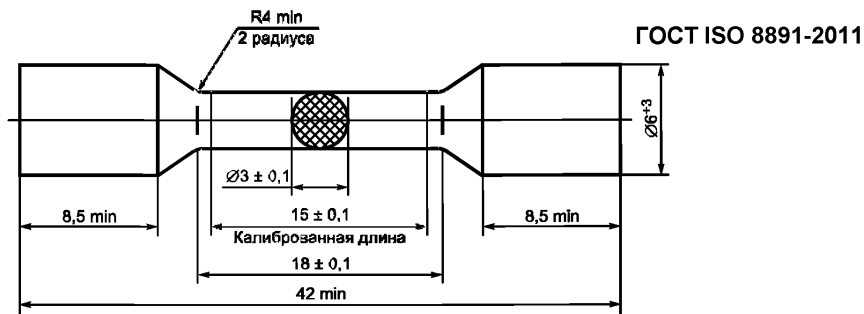
Рисунок 2 — Образец с удлиненной головкой
