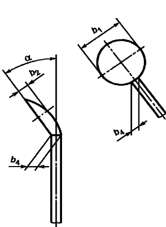
Рисунок 1 – Форма А: прямая
