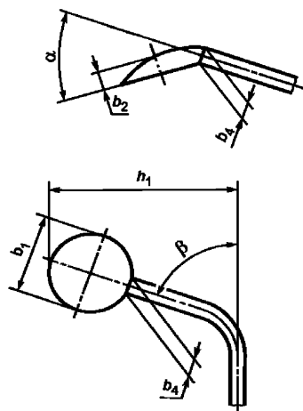
Рисунок 2 – Форма В: изогнута под углом
