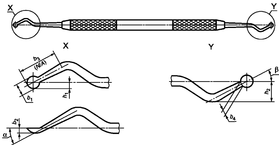
Рисунок 3 – Форма C: с двойным изгибом
