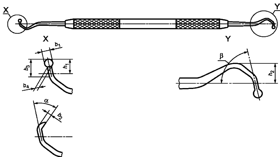
Рисунок 4 — Форма D: со сложным изгибом
