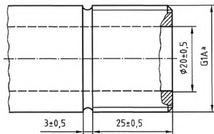
Рисунок 2 – Пример контрольного соединителя для ввода измерителя температуры
