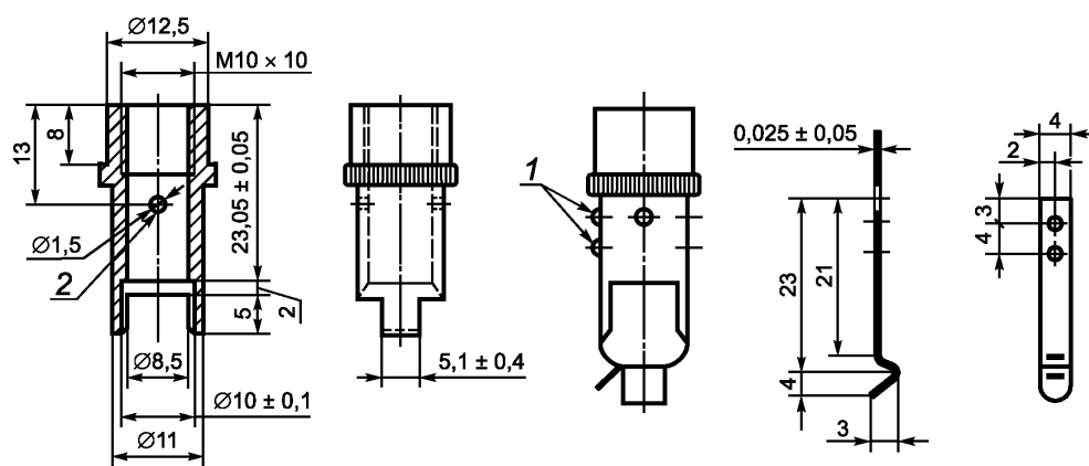
1 — заклепки или винты; 2 — отверстие
