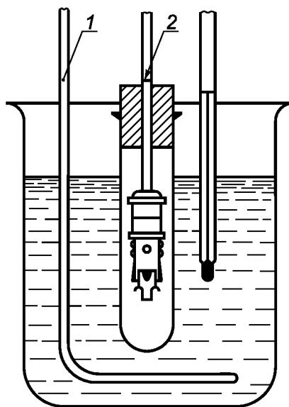
1 — мешалка; 2 — линия погружения
