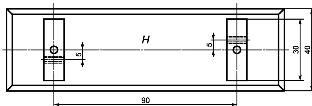
б) Плавкая вставка для поверхностного монтажа (схема печатной платы сверху)
