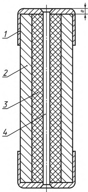
1 — колпачок; 2 — керамический корпус; 3 — наполнитель; 4 — плавкий элемент
