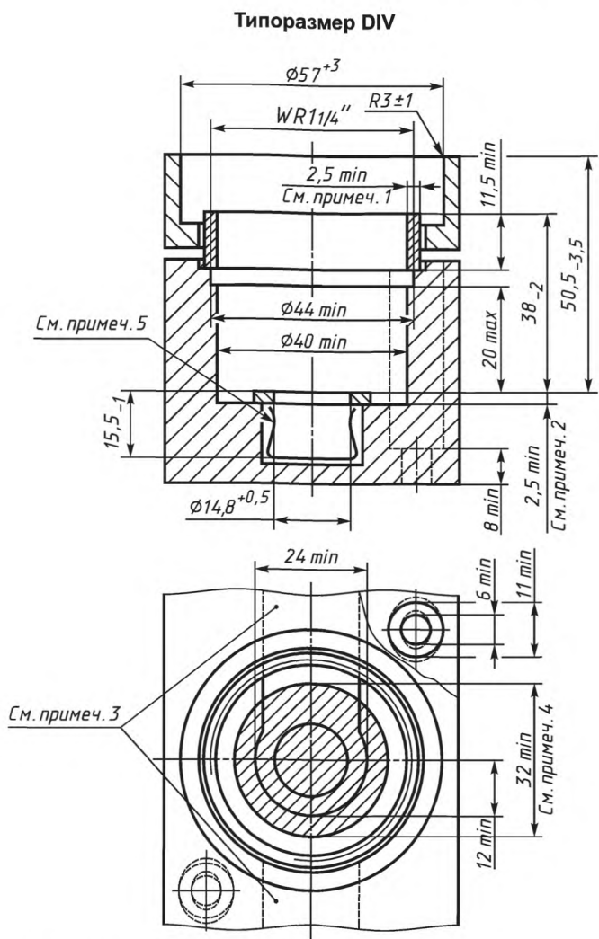
Рисунки не определяют конструкцию, а предназначены только для указания размеров. Изоляционные части — из керамического или другого материала с достаточной теплостойкостью.
