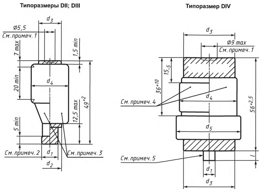
Рисунки не определяют конструкцию, а предназначены только для указания размеров. Заштрихованы контактные площадки. Корпус плавкой вставки — из керамического материала.
