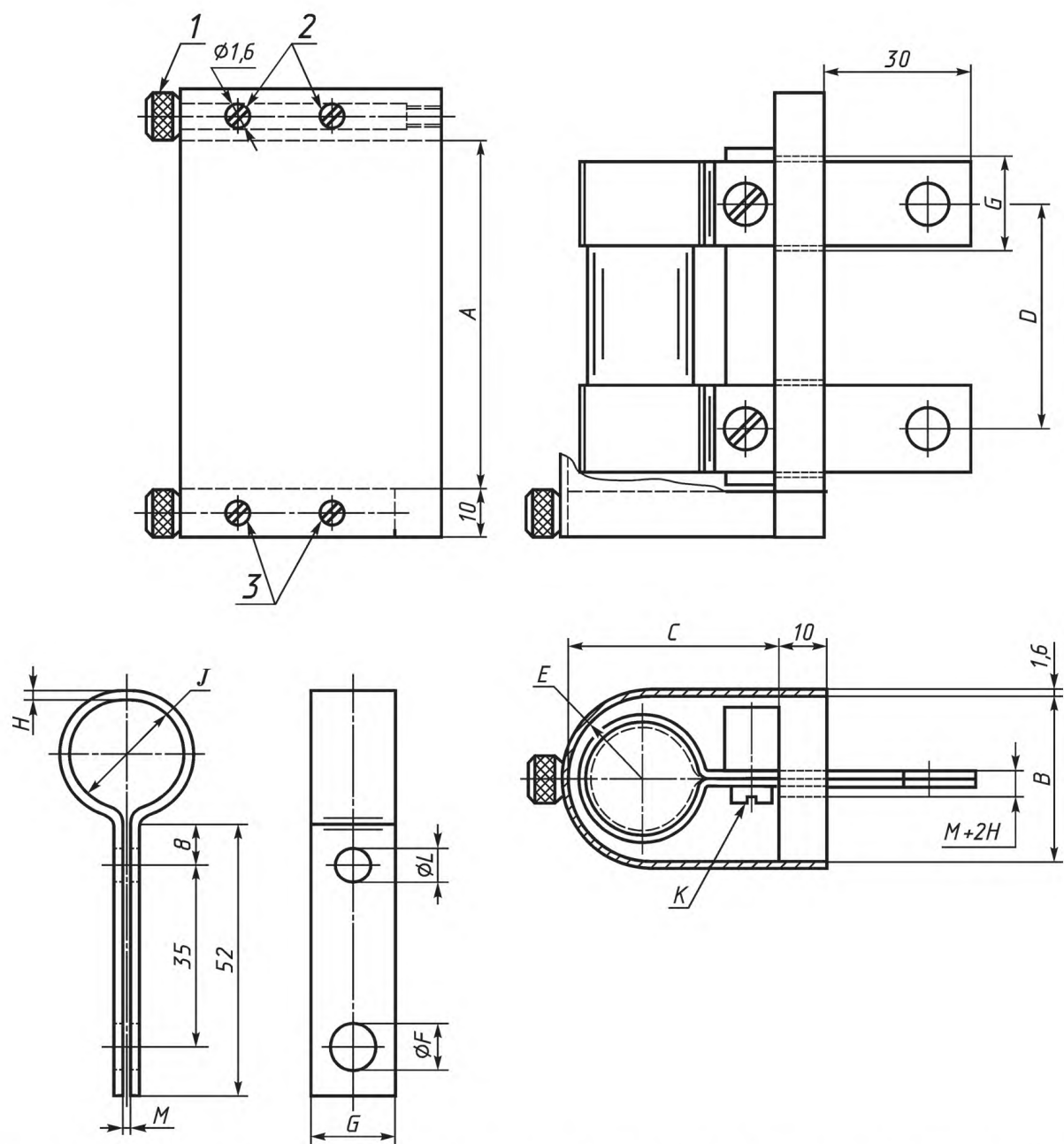
1 — винт, удерживающий крышку; 2 — отверстия в зажимных концах для датчиков измерения потерь мощности; 3 — зажимные концы, присоединенные к крышке; K — винт; H — толщина; J — внутренний диаметр; E — радиус; A, B, C — размеры внутренней части крышки
