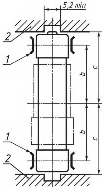
Контакты на цилиндрических поверхностях плавких вставок
