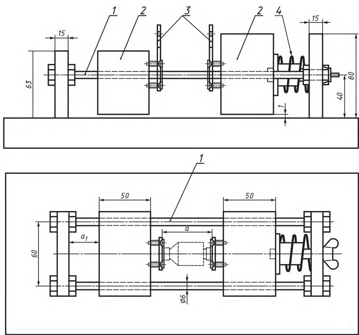
1 — металлический стержень диаметром 6 мм; 2 — изоляционный материал; 3 — участки контактов, покрытые слоем серебра; 4 — стальная пружина; a — см. на рисунке 3b; a 1 — расстояние для регулировки контактного усилия
