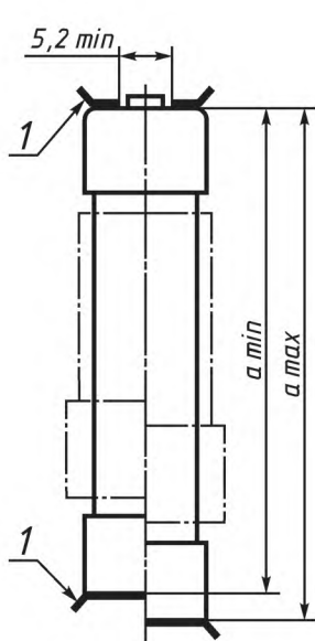
Контакты на торцевых поверхностях плавких вставок
