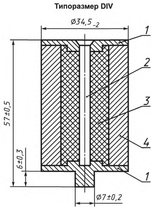
Рисунок 2 — Макетные плавкие вставки, соответствующие 8.3 и 8.9.1.1
