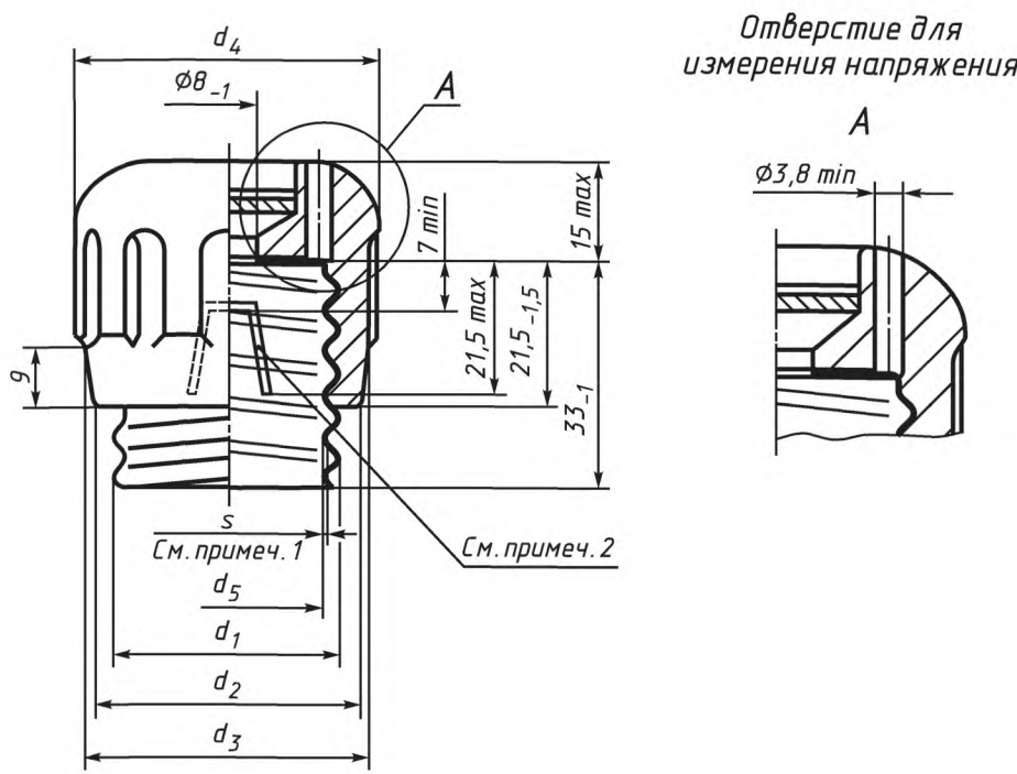
Рисунки не определяют конструкцию, а предназначены только для указания размеров. Изоляционные части — из керамического или другого материала с достаточной теплостойкостью.
