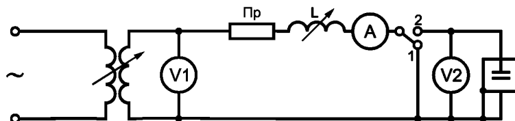
Пр — тугоплавкий предохранитель; L — регулируемая катушка индуктивности; V1 и V2 — вольтметры; A — амперметр
