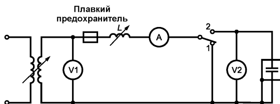
Рисунок 2 — Испытательная установка для разрушающего испытания переменным напряжением
