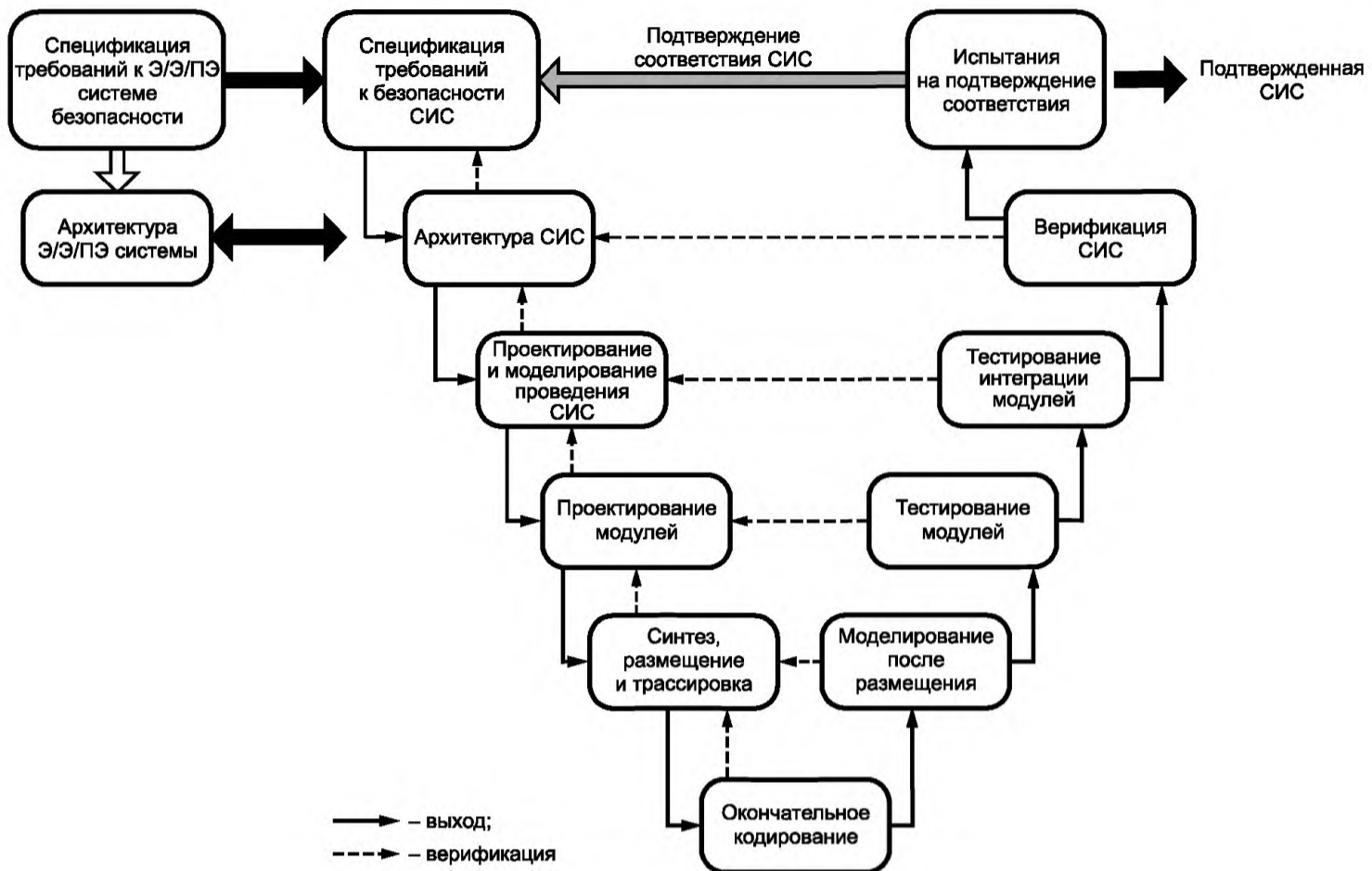
Рисунок 3 — Структура жизненного цикла разработки СИС (V-модель)
