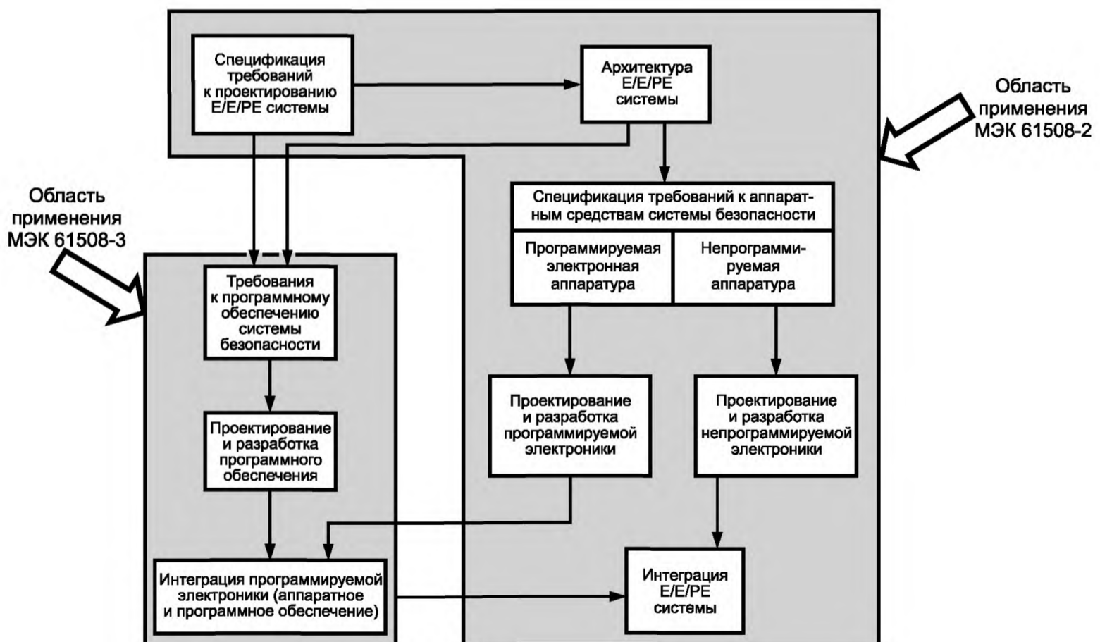
Рисунок 4 — Взаимосвязь и области применения МЭК 61508-2 и МЭК 61508-3
