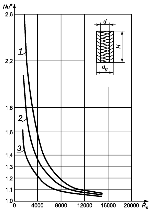
Рисунок А.5 — Диаграмма для теплоизоляционной системы общей толщиной d_g = 0,30 м
