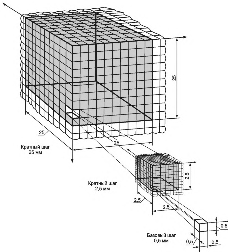
Рисунок 14 — Модульная сетка
