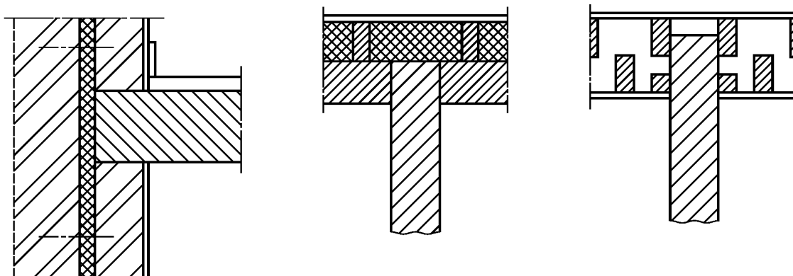
Рисунок Е.4 — Примеры жесткого Т-образного соединения
