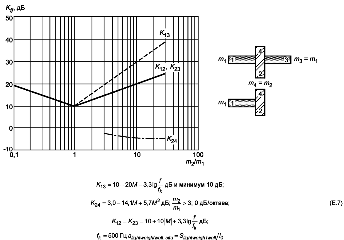
Рисунок Е.9 — Соединение легкой двухслойной стены и однородных элементов
