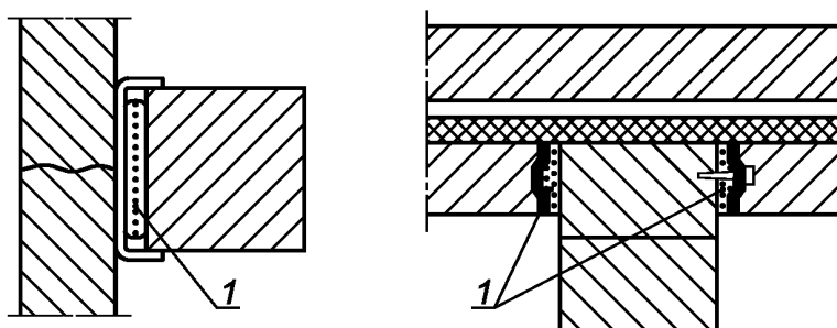
Рисунок Е.5 — Соединение со стеной через упругие прослойки
