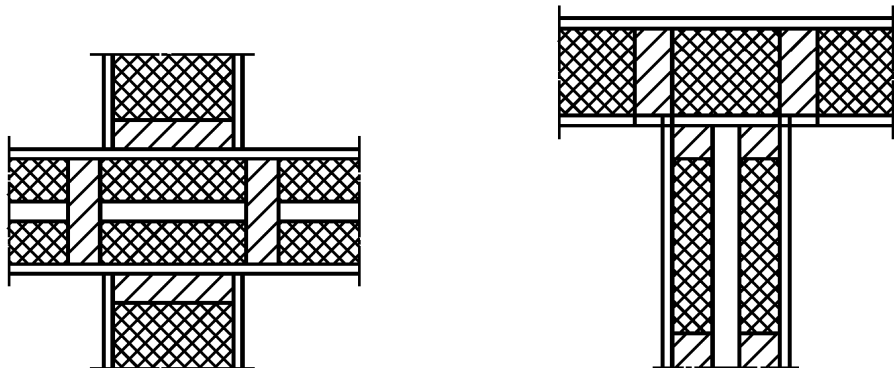
Рисунок Е.12 — Примеры соединений легкого элемента с двухслойными стенами
