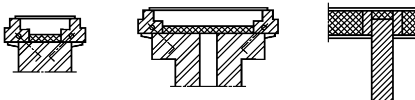
Рисунок Е. 8 — Примеры соединений легкого фасада
