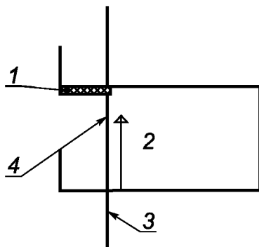
1 — звукопоглощающий материал; 2 — высота визирной линии; 3 — плоскость фасада; 4 — источник шума
