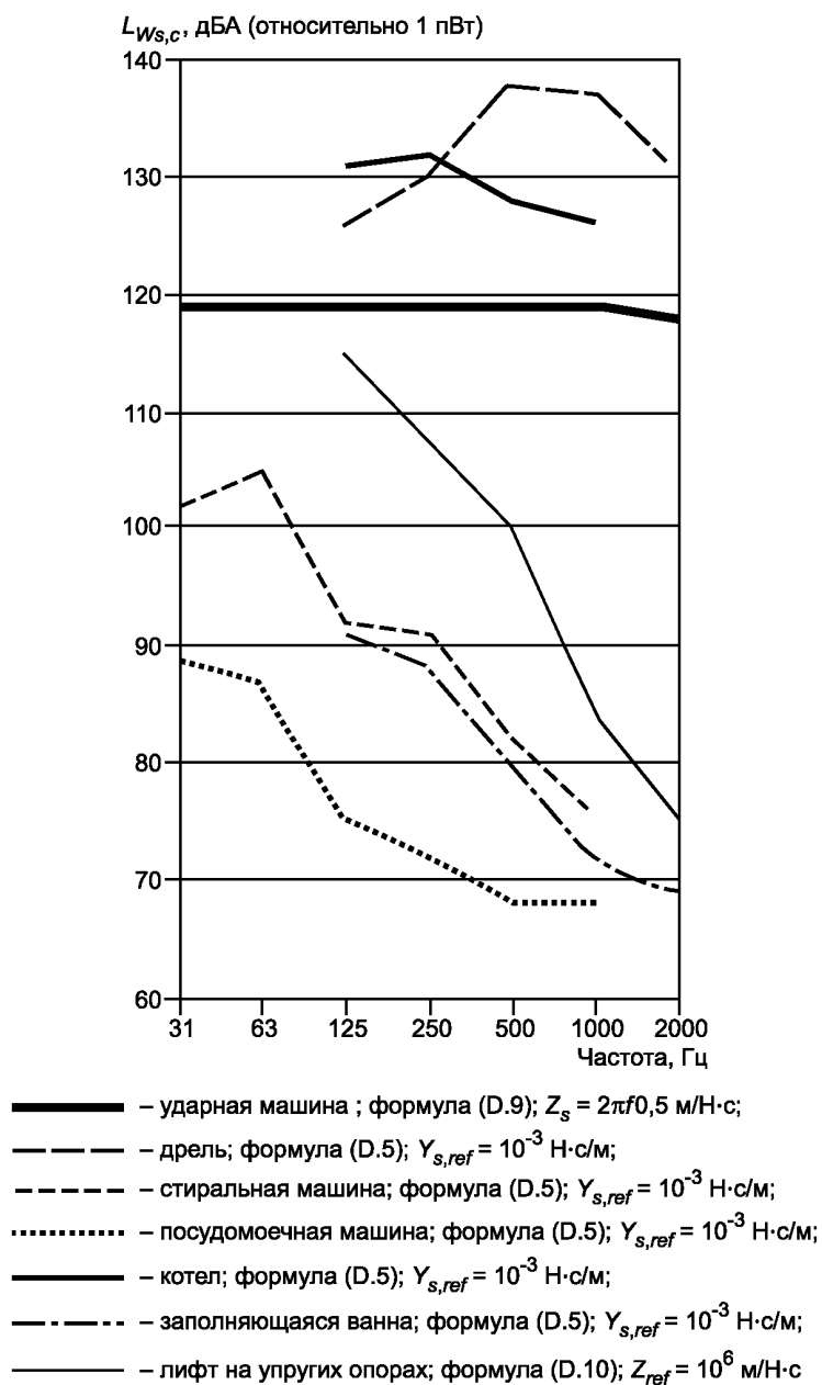
Рисунок D.4 — Зависимости от частоты уровня характеристической мощности некоторых источников структурного шума, определенные с помощью формул (D.5), (D.9) и (D.10) на основании результатов измерений силы или скорости вибрации [11], [17], [18]
