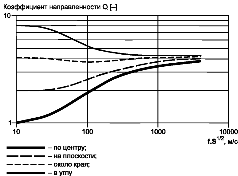
Рисунок Е.1 — Коэффициент направленности излучения Q отверстий в различных местах помещения для излучения под углом 45^\circ как функция их площади и частоты (комбинированный эффект влияния направленности излучения отверстий вблизи отражающих поверхностей по [1])
