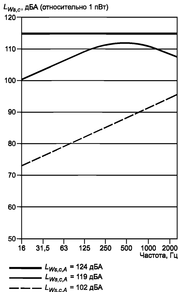
Рисунок D.3 — Мощность структурного шума ударной машины: характеристическая мощность источника, переданная мощность для деревянного и бетонного пола
