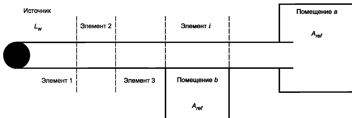
Рисунок 1 — Звукопередача от источника воздушного шума по зданию через систему воздуховодов в приемные помещения ( a и b )
