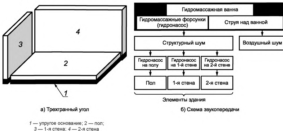
Рисунок 7 — Звукопередача шума от гидромассажной ванны
