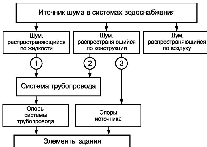
Рисунок 4 — Пути звукопередачи от источников шума в системах водоснабжения
