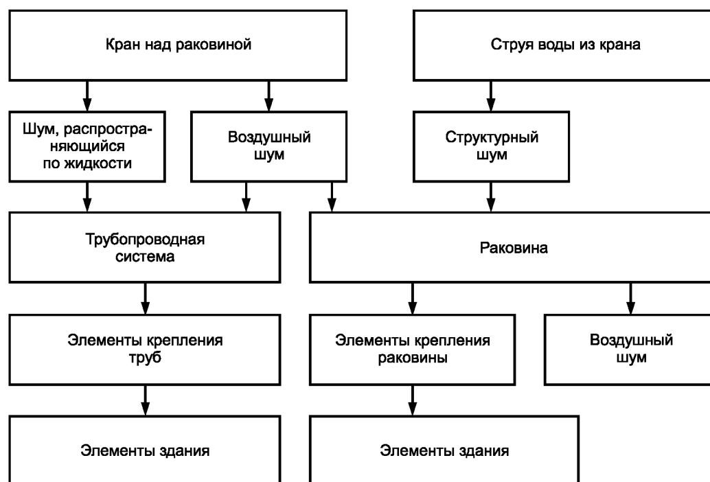
Рисунок 5 — Пути звукопередачи от крана над раковиной
