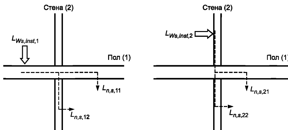
Рисунок 1.3 — Побочные пути косвенной звукопередачи
