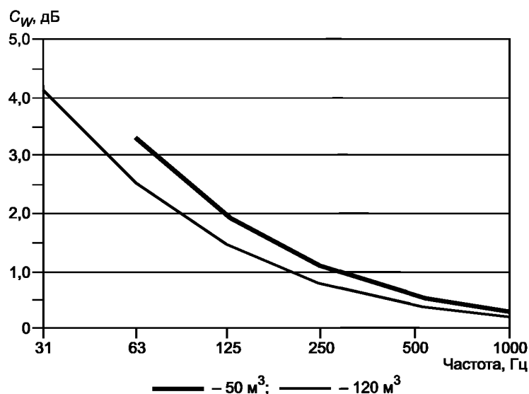
Рисунок G.1 — Пример зависимости поправки Уотерхауса от частоты для двух высоких прямоугольных помещений нижнего этажа
