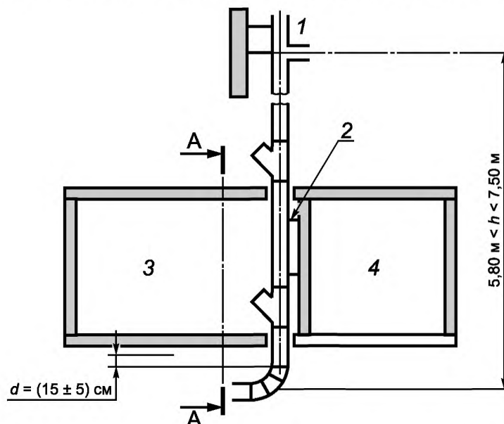
1 — входное отверстие; 2 — крепление к разделительной стене; 3 — помещение источника; 4 — приемное помещение
