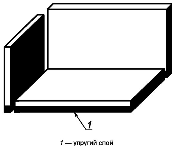
Рисунок D.1 — Схематичное изображение испытательного стенда с тремя плитами
