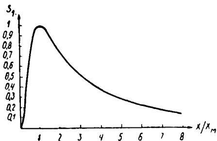
РИС. 7. ГРАФИК ДЛЯ ОПРЕДЕЛЕНИЯ ЗНАЧЕНИЙ БЕЗРАЗМЕРНОГО КОЭФФИЦИЕНТА s_1 (ПРИ \frac{x}{x_m} < 8 )
