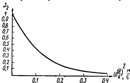
РИС. 9. ГРАФИК ДЛЯ ОПРЕДЕЛЕНИЯ ЗНАЧЕНИЙ БЕЗРАЗМЕРНОГО КОЭФ. ФИЦИЕНТА s_2
