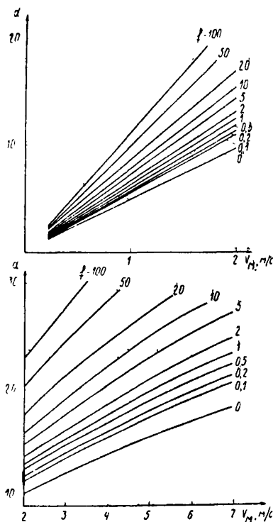
РИС. 5. ГРАФИКИ ДЛЯ ОПРЕДЕЛЕНИЯ ЗНАЧЕНИЙ БЕЗРАЗМЕРНОГО КОЭФФИЦИЕНТА a
