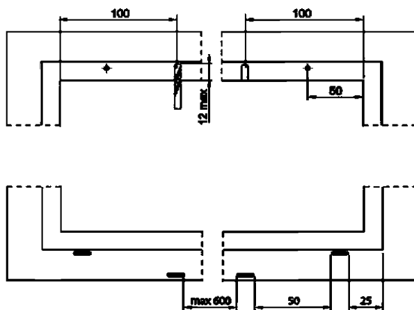
Рисунок Г.9 – Схема расположения водосливных отверстий
