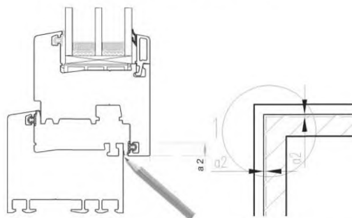
Рисунок. Г.4а – Нанесение контрольных меток
