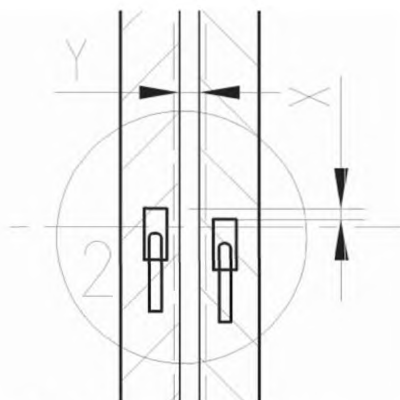
Рисунок Г.3 – Сопряжение смежных створок СПК
