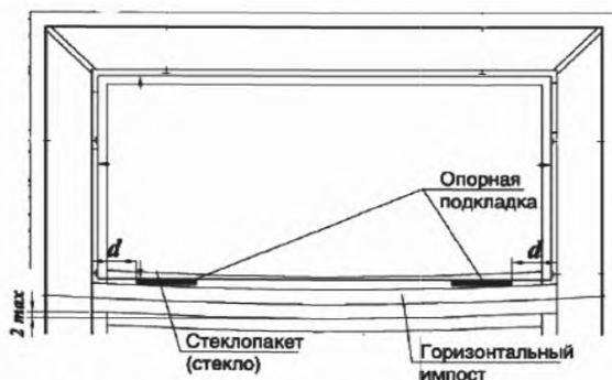
Рисунок Г.7 – Схема деформации импоста
