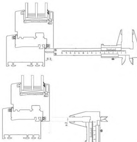
Рисунок. Г.4б – Замер контрольных меток
