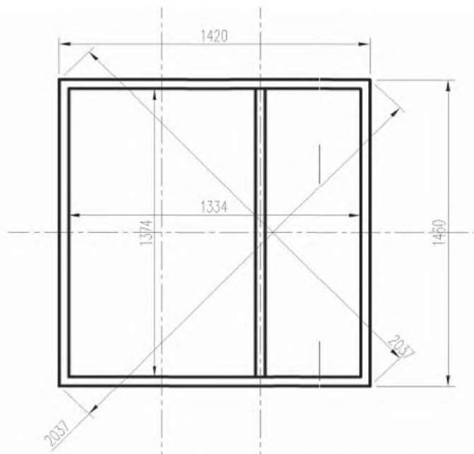
Рисунок Г.1 Оценка геометрических размеров СПК
