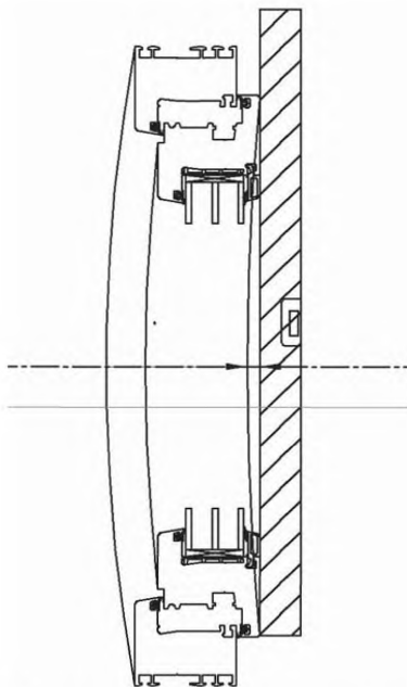
Рисунок Г.8 – Форма прогиба основных профилей
