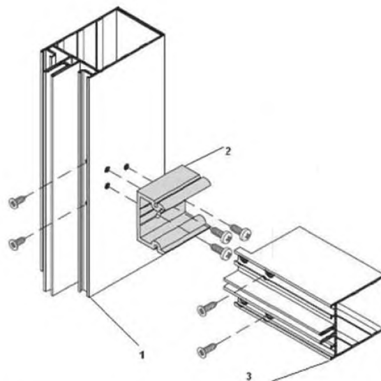
Рисунок 5.3 – Установка ригеля
