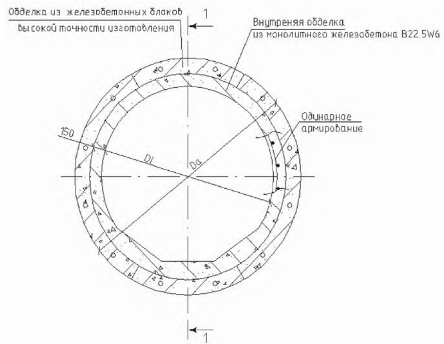
Рисунок Г.2 – Конструкция канализационного тоннеля тип II
