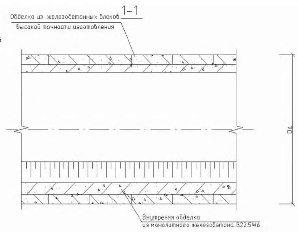
Рисунок Г.2 – Конструкция канализационного тоннеля тип II
