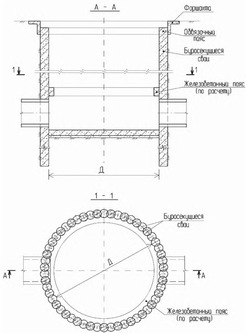
Рисунок 10.5 – Круглый шахтный ствол, сооружаемый методом «стена в грунте» из буресекущих свай
