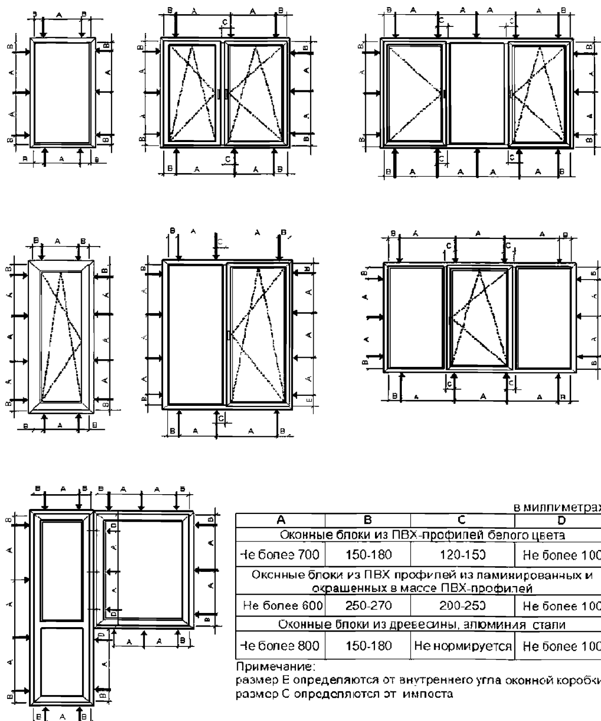
Рисунок Ж.3 – Примеры расположения точек крепления некоторых вариантов оконных блоков
