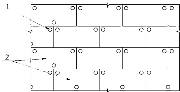
Схема установки внешнего слоя.
