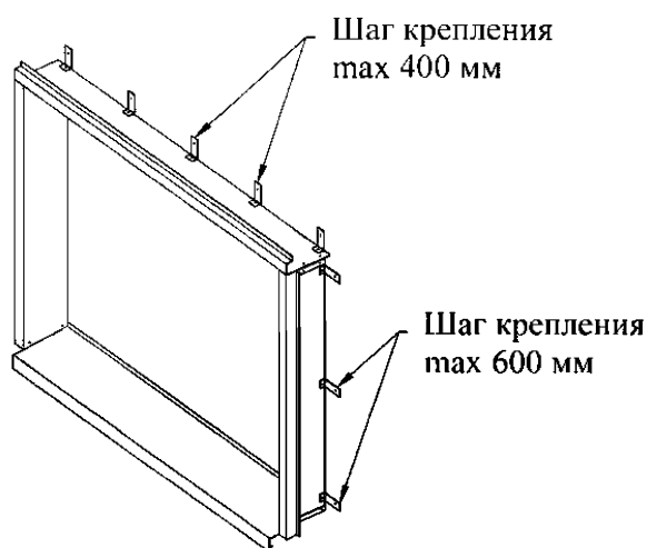
Противопожарный короб закрытого типа (варианты)
