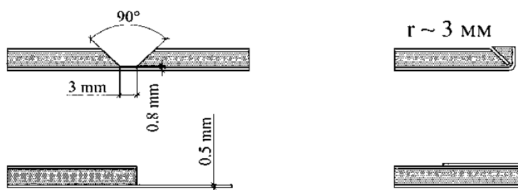
Рисунок 6 – Виды фрезеровок
