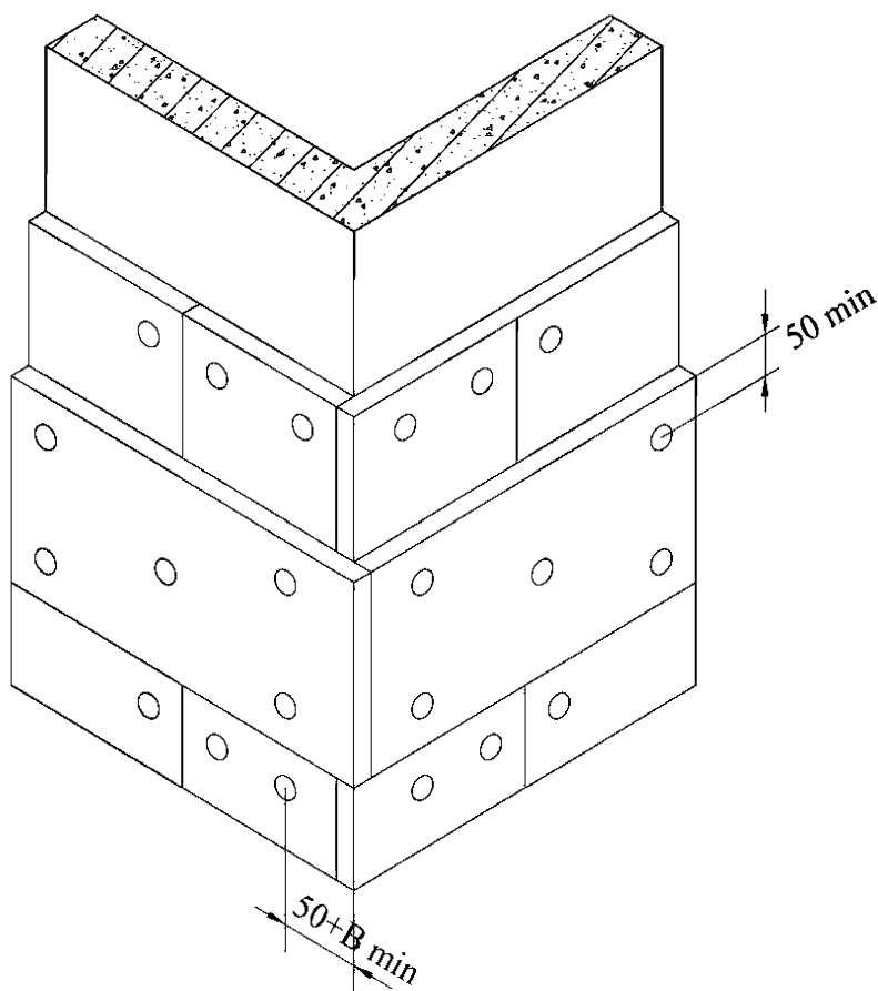
Рисунок 1 – Схема крепления двухслойного утеплителя на углу здания
