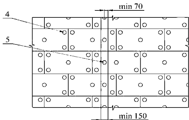
Схема установки ветрогидрозащитной мембраны.
