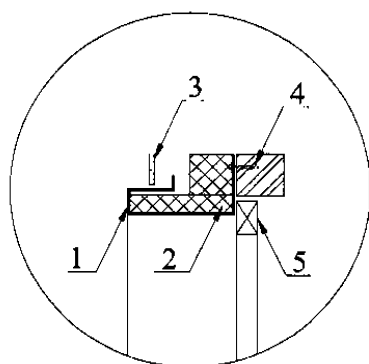
Противопожарный короб открытого типа
