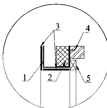
Противопожарный короб закрытого типа (варианты)
